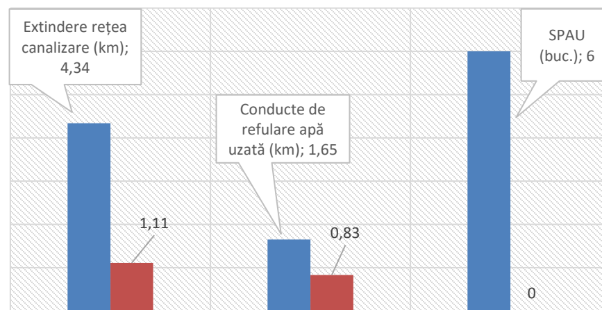
Progres lucrări canalizare CL6
